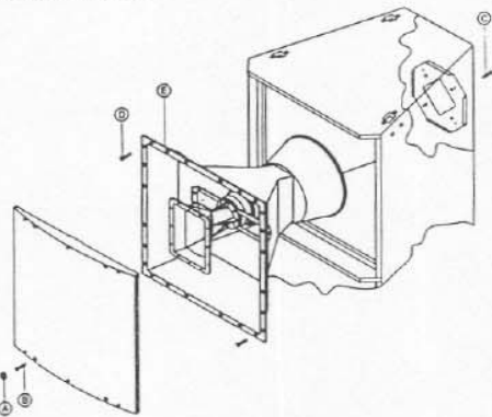
FIGURE 5 — Module Rotation
